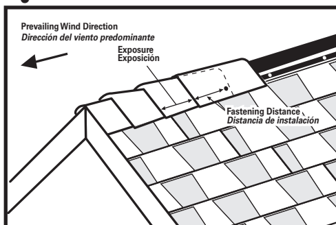
Fig. 8 Hip & Ridge Application Instalación de tejas para caballetes y cumbres
